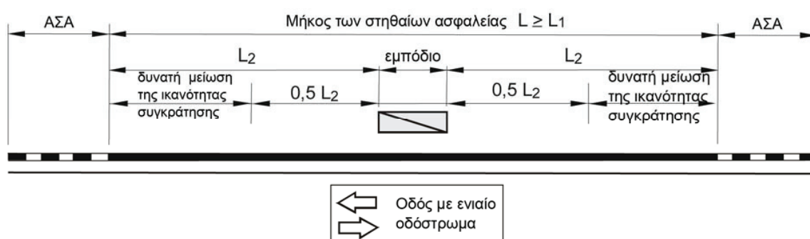
Σχ. 14α: Μήκη των στηθαίων ασφαλείας σε οδούς με ενιαίο οδόστρωμα
